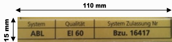
Brandschutz Kennzeichnungsschild Aluminium eloxiert
