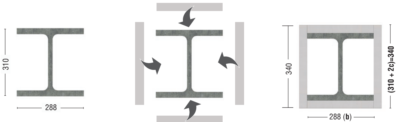
A1 COREX Abmessungen
