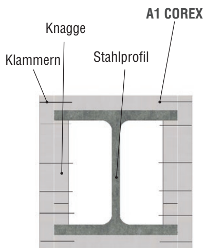
Einlagig A1 COREX
