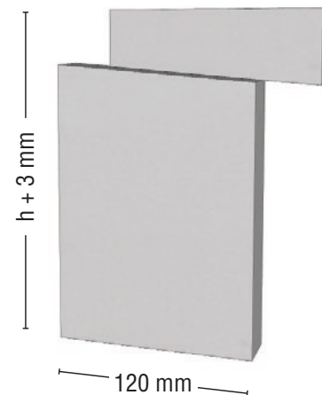
Abmessungen der Knagge
