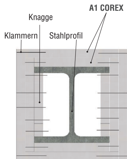
Zweilagig A1 COREX
