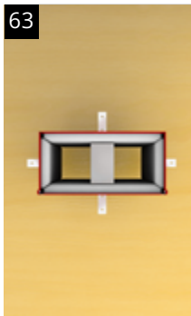
63 Prüfen Mitgelieferten Hartschaumblock mittig anordnen, oben und unten die Schaumplatten. Dadurch kein Verformen der FST-Kombibox beim Vergießen des Ortbetons.
