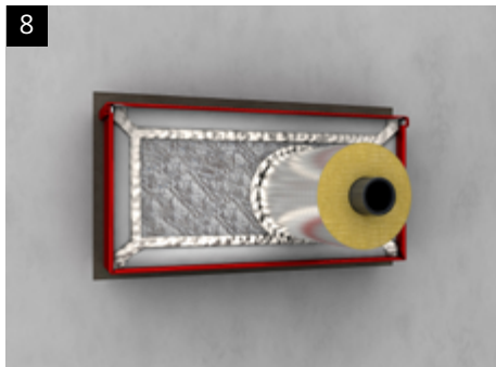
(Edel)Stahl-, Guss-Rohre d_a \leq 60,3 mm (DN 50) mit beidseitiger Streckenisolierung aus Mineralfaserrohr- schalen (Schmelzpunkt > 1.000 °C, L = 500 mm, d = 20 mm)
