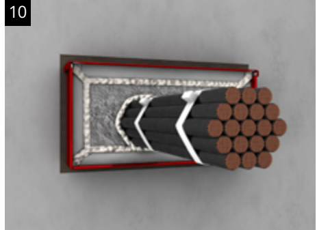
Kabelbündel d_a \leq 100 mm, parallel verlaufend, dicht gepackt und miteinander fest verschnürt, vernäht und verschweißt, max. Kabeleinzel- durchmesser 20 mm
