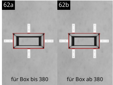
62a Winkel befestigen Winkel am Boxenrand andrücken. (Lieferumfang: 4 bis 6 Winkel je nach Boxengröße)
