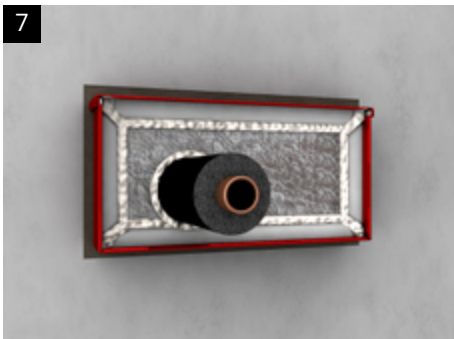
Kupferrohre d_a \leq 35 mm (DN 32) mit durchgehenden synth. Kautschukisolationen, d = 13 mm
