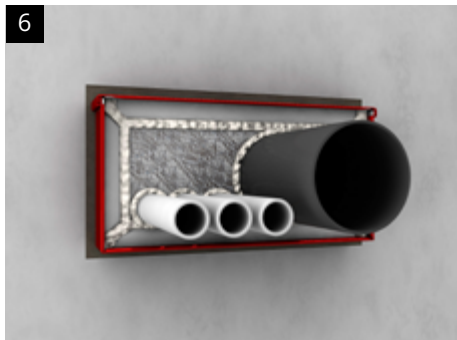
Kunststoffrohre PE-Rohre (nur Versorgungsrohre) bis d_a \leq 75 mm (DN 70) siehe aBG
